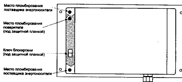
б) исполнение для щитового монтажа (вид сзади)
