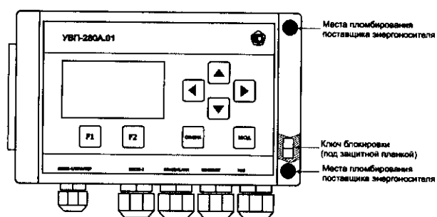
Рисунок 3. Места пломбирования вычислителей УВП-280А.01
