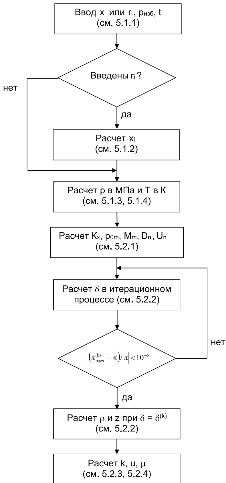
Рисунок 1 — Блок-схема расчета физических свойств природного газа
