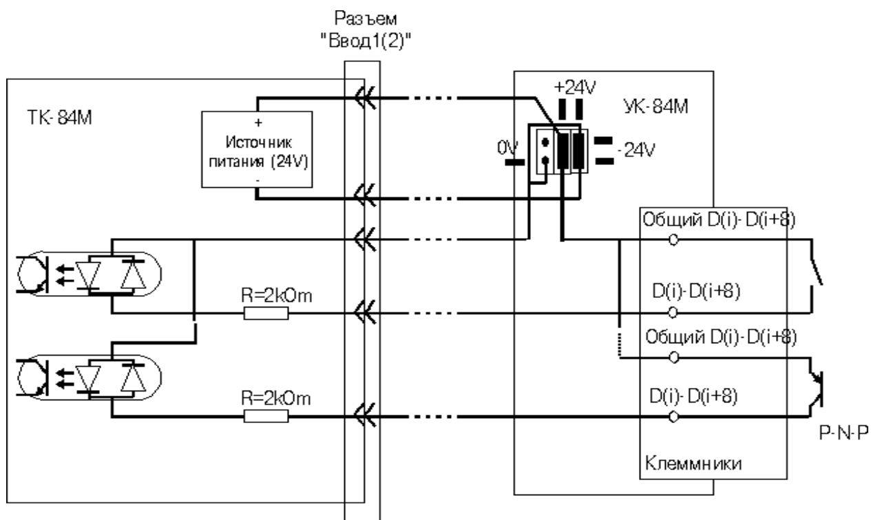
Рис.4 Схема подключения дискретных датчиков с питанием +24В
