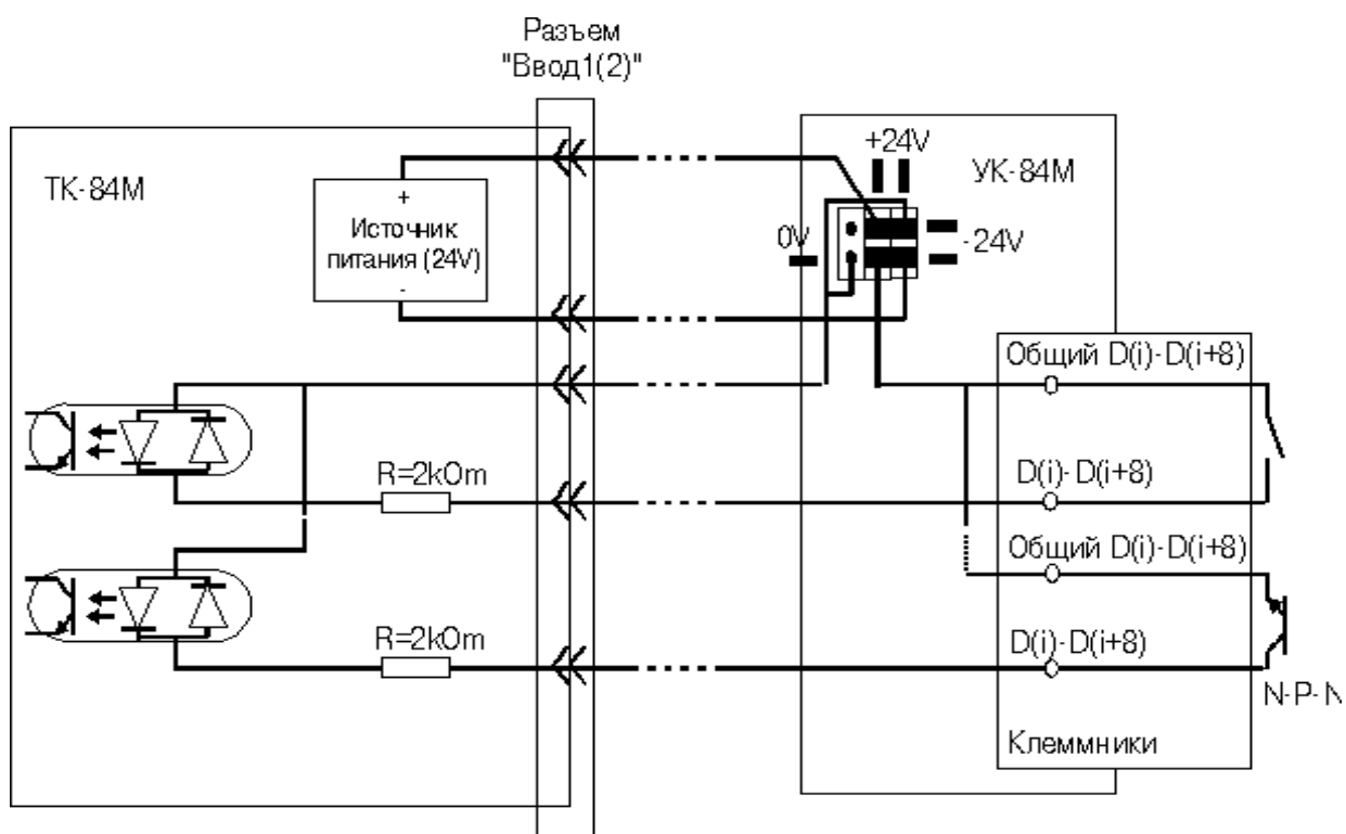
Рис.4 Схема подключения дискретных датчиков с питанием +24В
